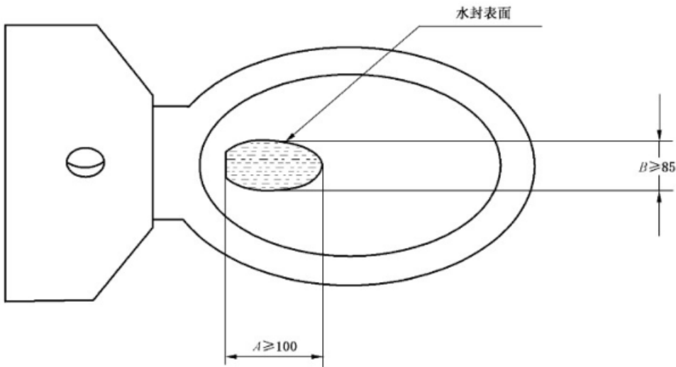
图 1 水封表面面积测试示意图
